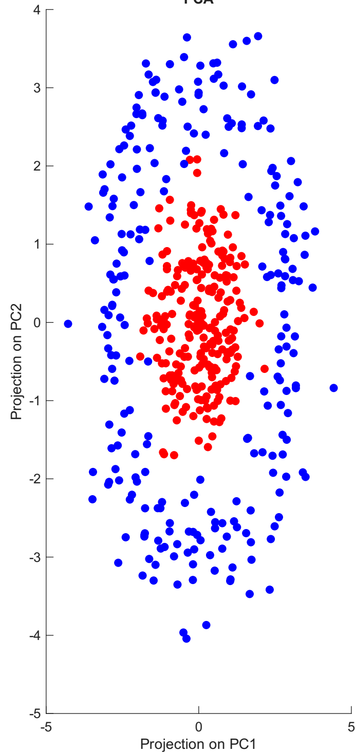
PCA
